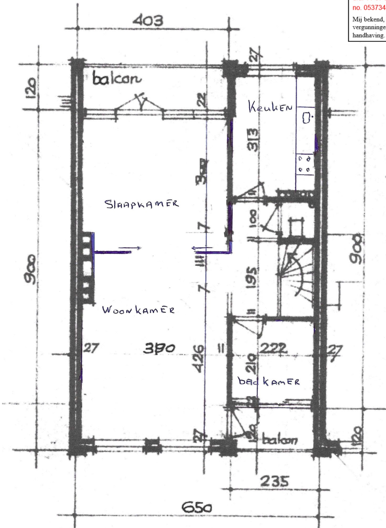
2 e verdiepingplan.
