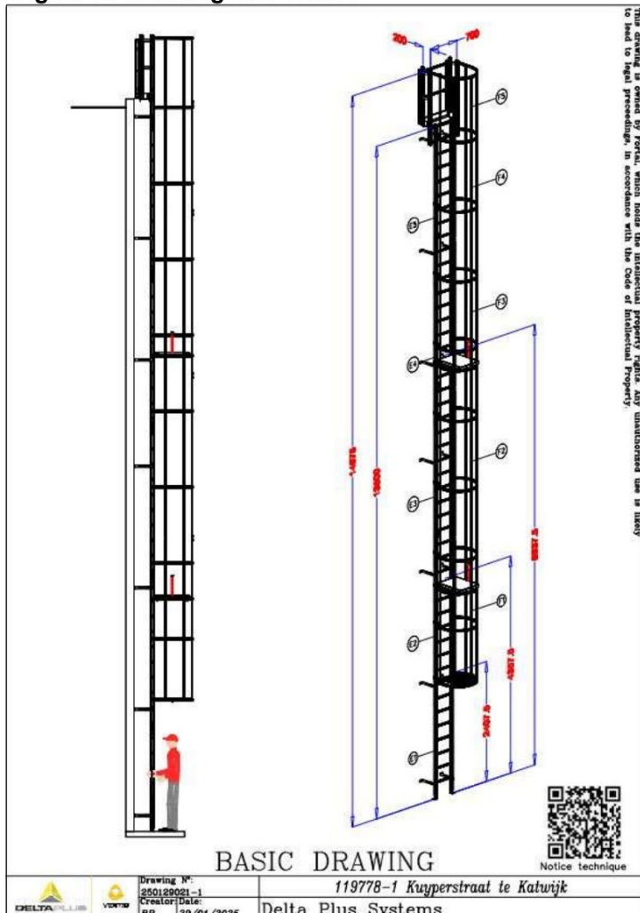
Figuur 2: Tekening kooiladder.
