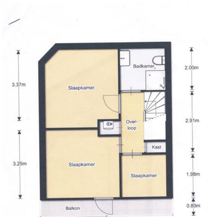
2 verdieping
