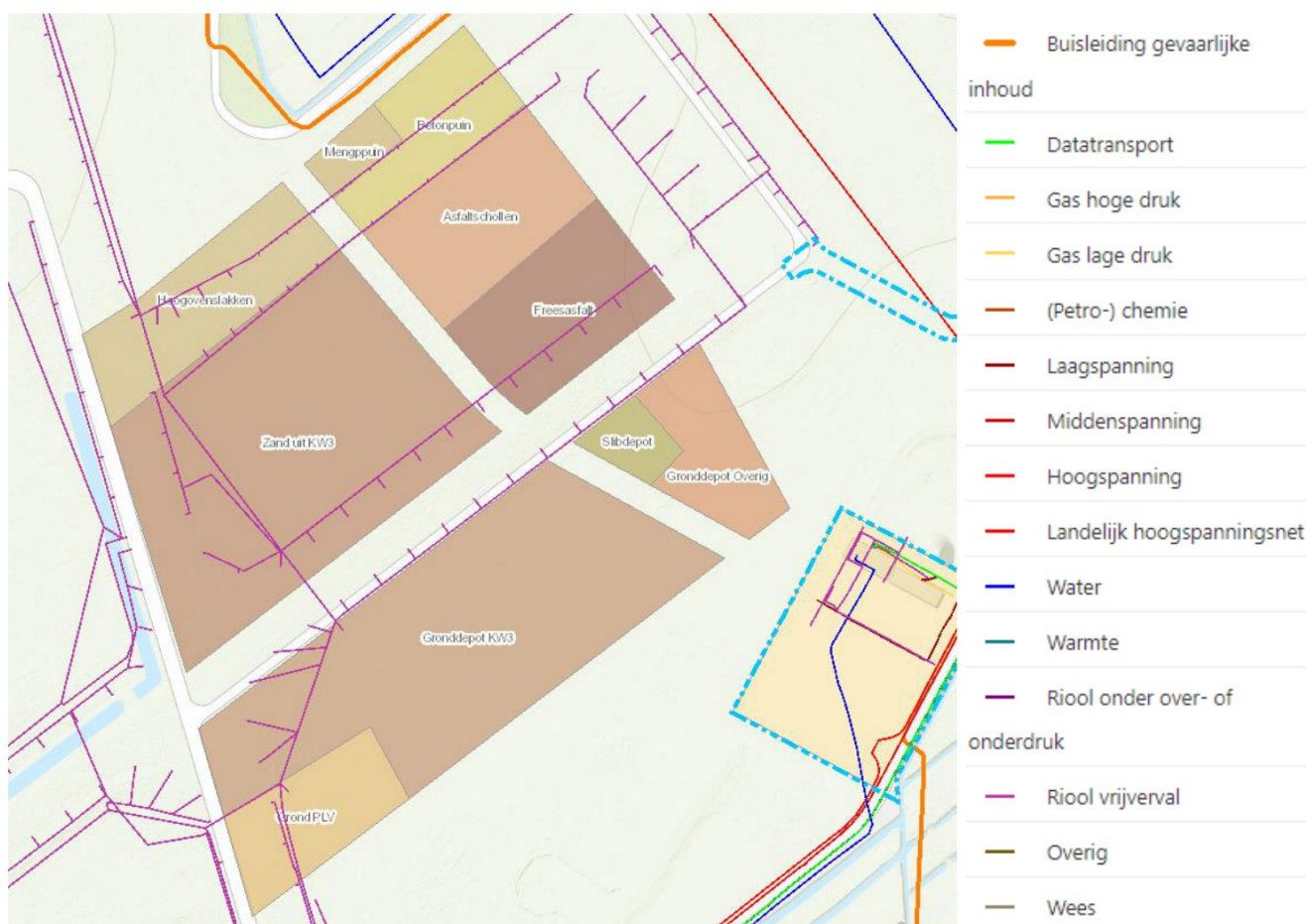
Figuur 2 Kabels- en leidingen depot PLV
