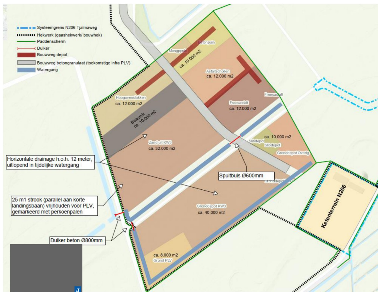
Figuur 6 Overzichtstekening depot PLV
