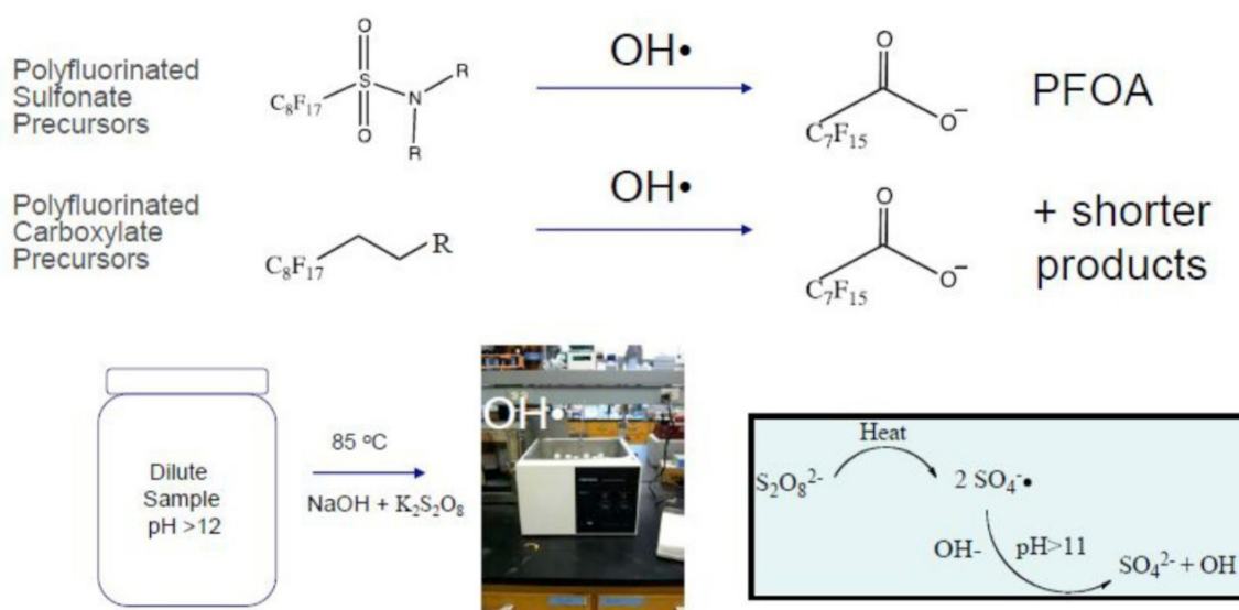
Afbeelding 2.5 Schematische weergave principe TOP-analyse
