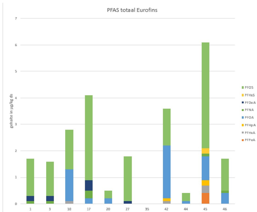
Abbeelding 4.7 Samenstelling PFAS componenten per monsternamelocatie Eurofins
