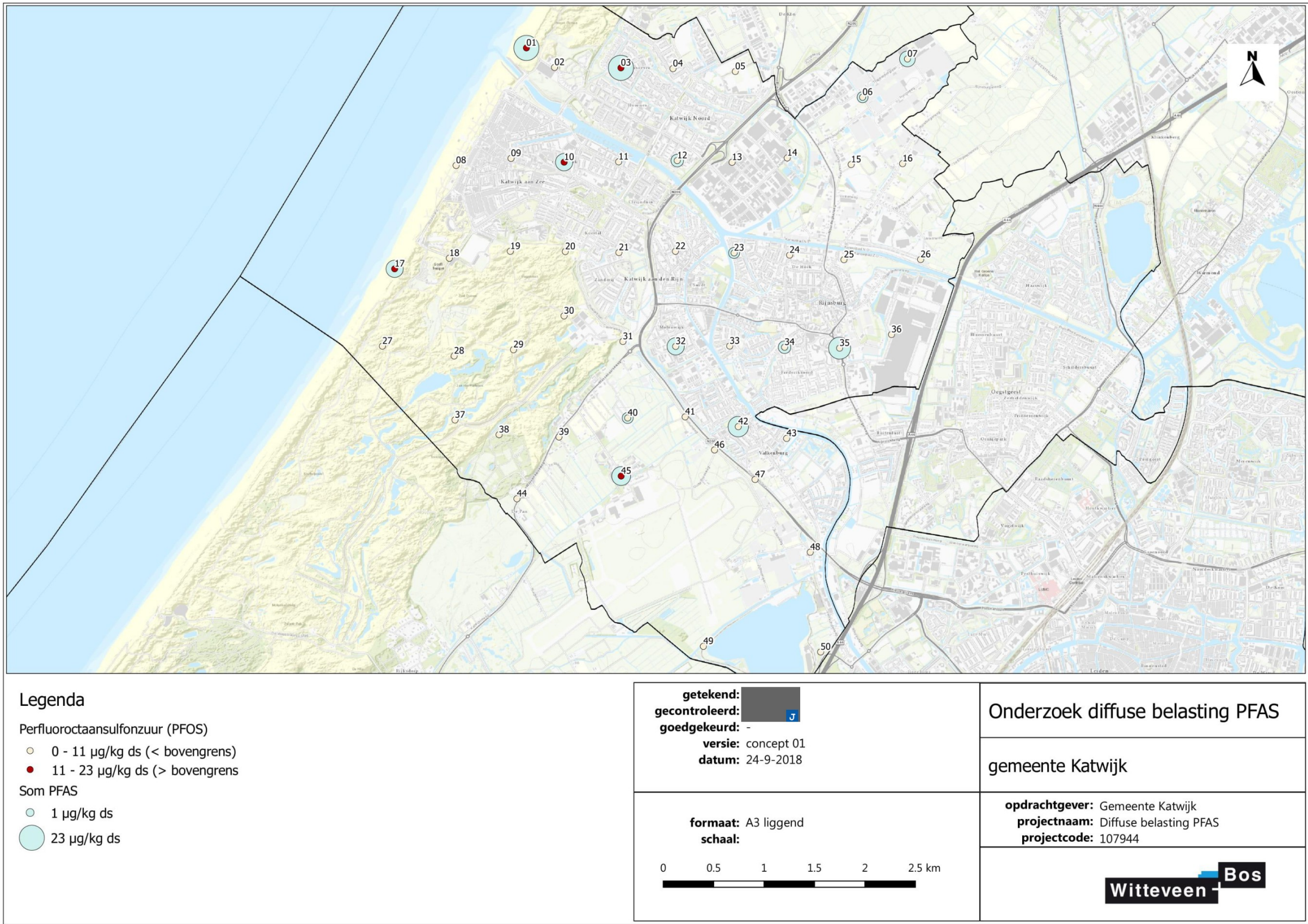
Afbeelding 3.1 PFOS overschrijdingen
