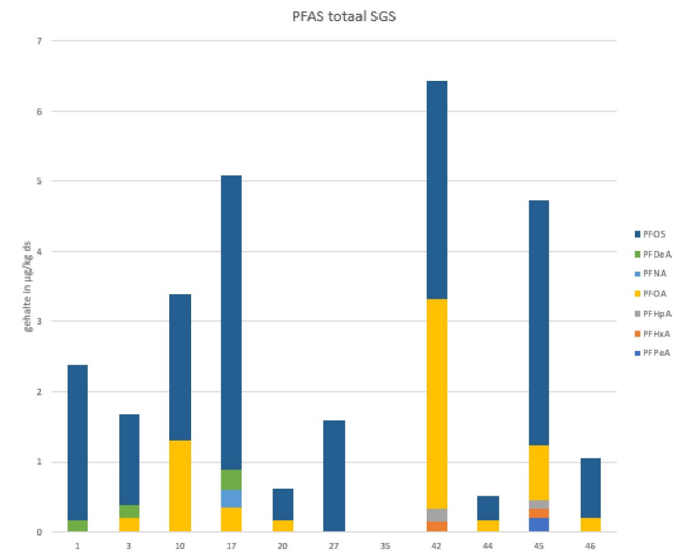
Abbeelding 4.6 Samenstelling PFAS componenten per monsternamelocatie SGS
